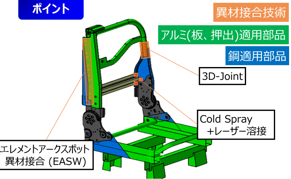
マルチマテリアル(MM)シートフレームコンセプト
